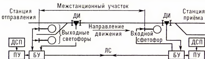
Схема релейной полуволновой блокировки: ПУ — пульт управления; БУ — блокирующие устройства; ЛС — линия связи; ДИ — датчики информации; ДСП — датчик путевого светофора.
